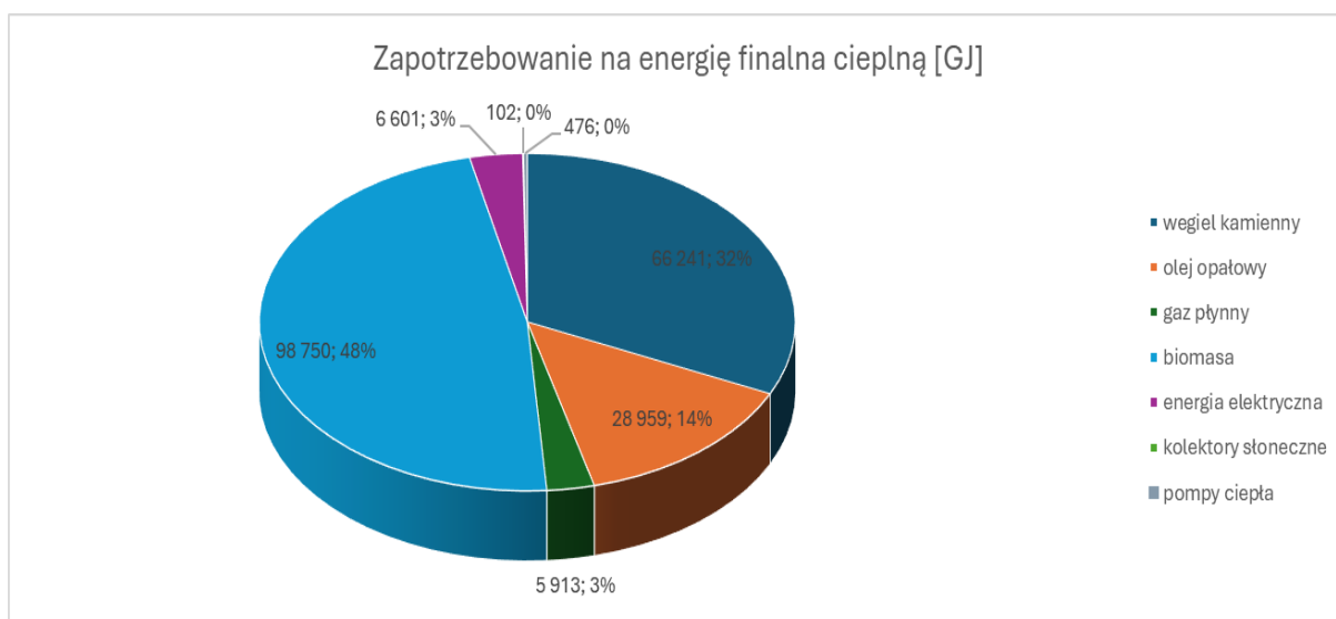
Rys. 14 Zapotrzebowanie na energię finalną cieplną w gminie Drawsko
